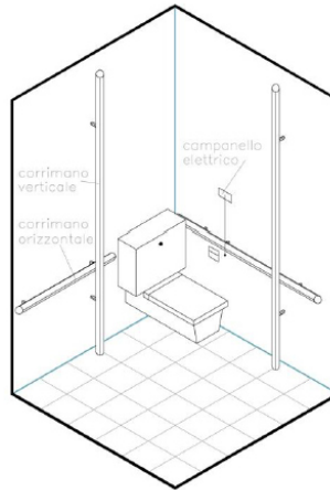
Vista assometrica
