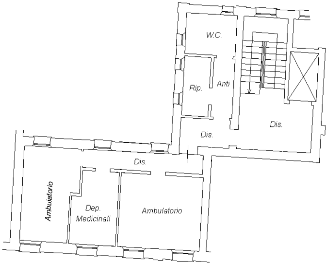
PIANO PRIMO H=2.77
